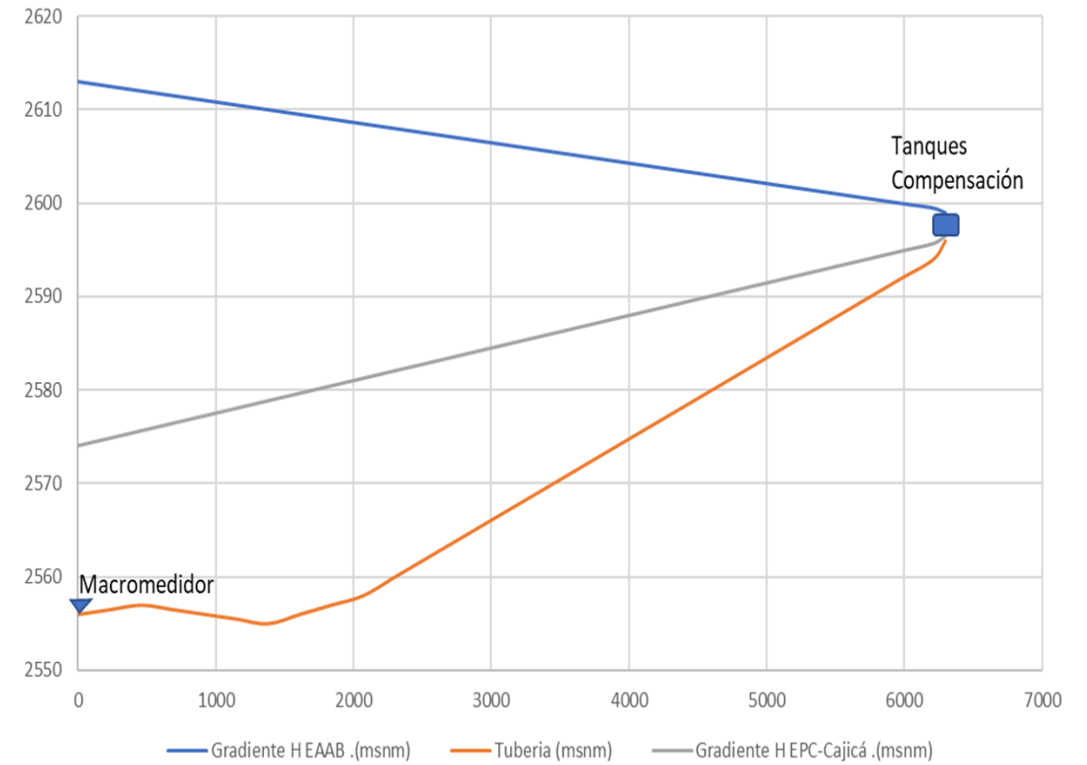
Esquema Hidraulico Acueducto Tanque Occidental
