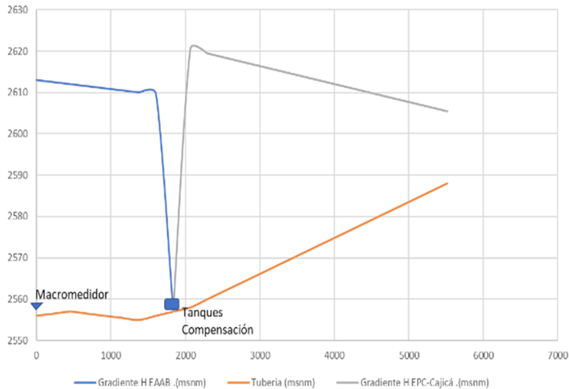
Esquema Hidraulico Acueducto Tanque Oriental
