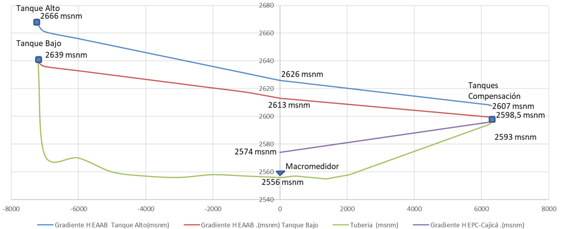
Esquema Hidraulico Acueducto Tanque Occidental
